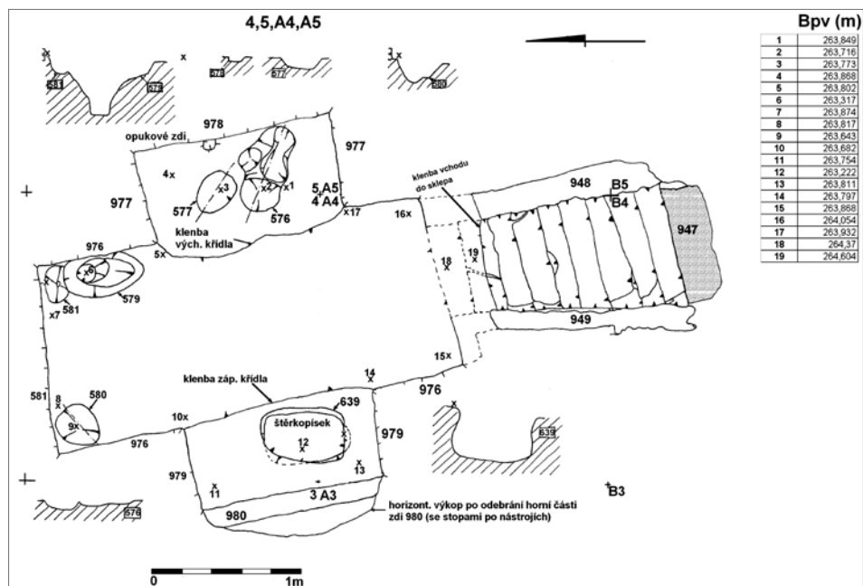
Obr. 8. Chrudim, Hradební ul. Půdorys druhého patra sklepa o křížovém půdorys s patrnými podzemními skříšemi. V západním výklenku je patrně odstranění části zazdívky z důvodu hledání skříše. Kresba P. Leidemann, digitalizace J. Musil. Abb. 8. Chrudim, Hradební-Gasse, Grundriss des zweiten Kellergeschosses mit kreuzförmigem Grundriss und erkennbaren unterirdischen Verstecken. In der westlichen Nische kann man die zwecks Suche des Verstecks erfolgte Entfernung eines Teils der Einmauerung erkennen. Zeichnung P. Leidemann, Digitalisierung J. Musil.
